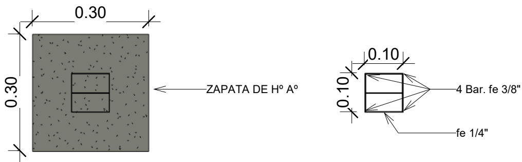
A DET. ANCLAJE 1 : 10
