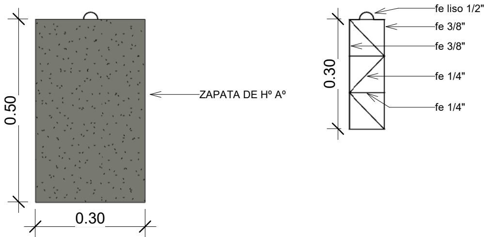
A DET. ANCLAJE 1 : 10
