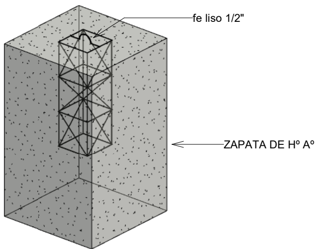
A2 VISTA ANCLAJE
