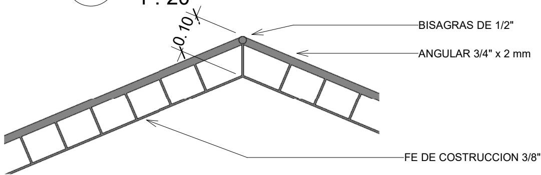
E DETALLE CERCHA 1 : 10
