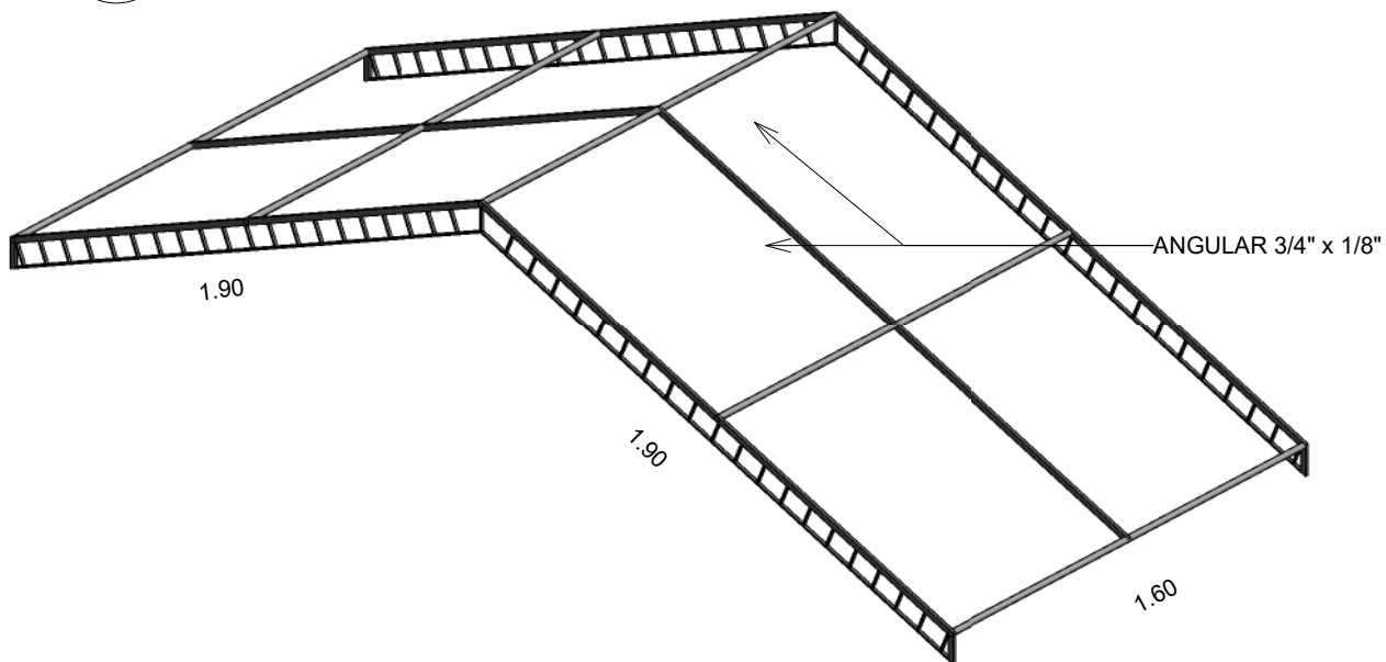
F ESTRUCTURA CUBIERTA
