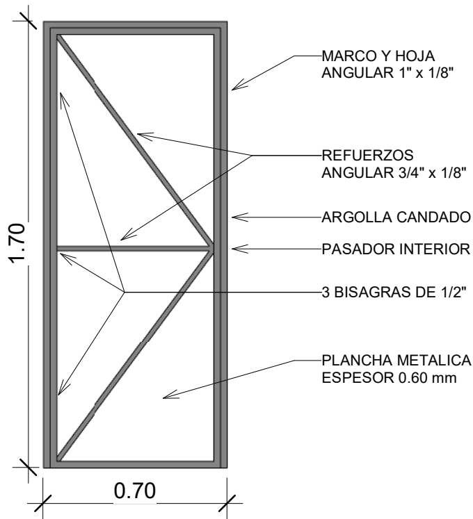
C DETALLE PUERTA 1 : 20
