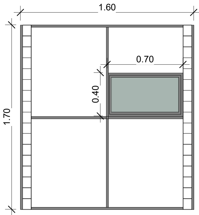
B LATERAL CON VENTANA 1 : 20
