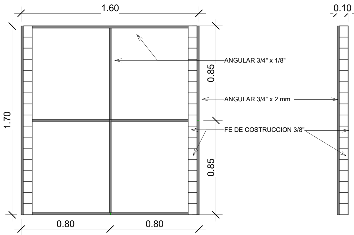
D LATERAL SIN VENTANA 1 : 20
