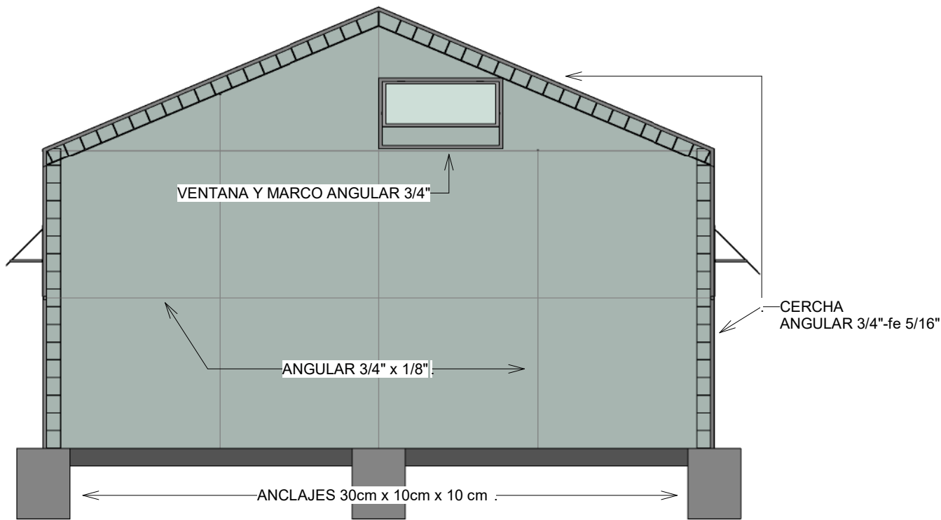
1 ELEVACION POSTERIOR 1 : 30
