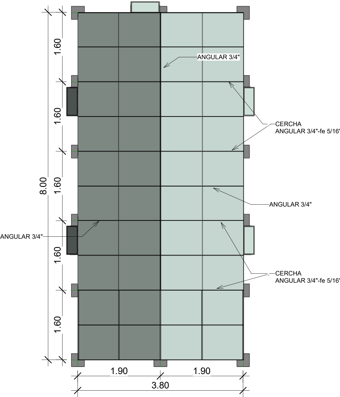
1 PLANO DE TECHOS 1 : 50
